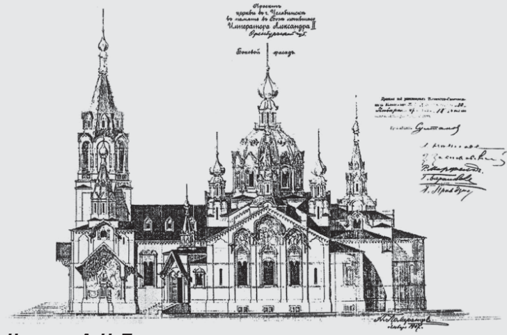
Чертеж А. Н. Померанцева.
